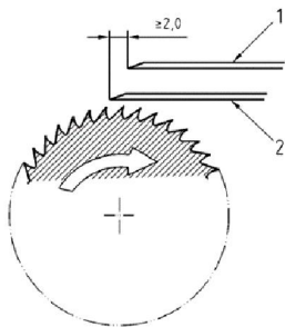
Figura 11 - Detalhe do dispositivo de lâmina dupla
